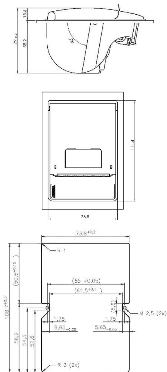
Abbildung 2: Abmessungen GeBE-MULDE Mini GPT-4352-60 (max. ø 60 mm Papierrolle) in mm
