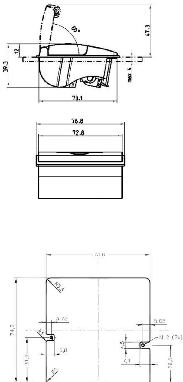
Abbildung 1: Abmessungen GeBE-MULDE Mini GPT-4352 (max. ø 31 mm Papierrolle) in mm
