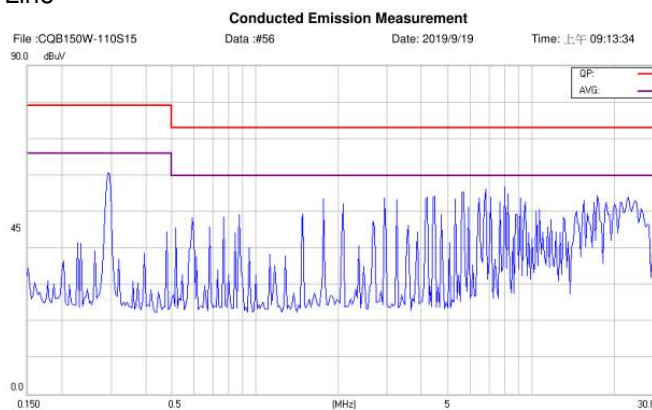
CQB150W-110S15-CMFC(D) Line
