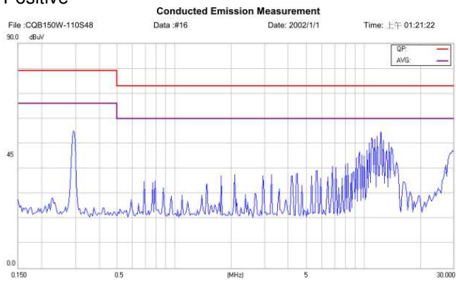
CQB150W-110S48-CMFC(D) Positive
