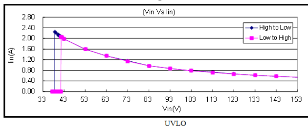
CQB150W-110SXX-CMFC(D) lin Vs Vin
