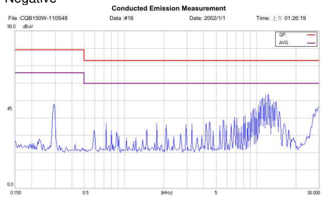
CQB150W-110S48-CMFC(D) Negative
