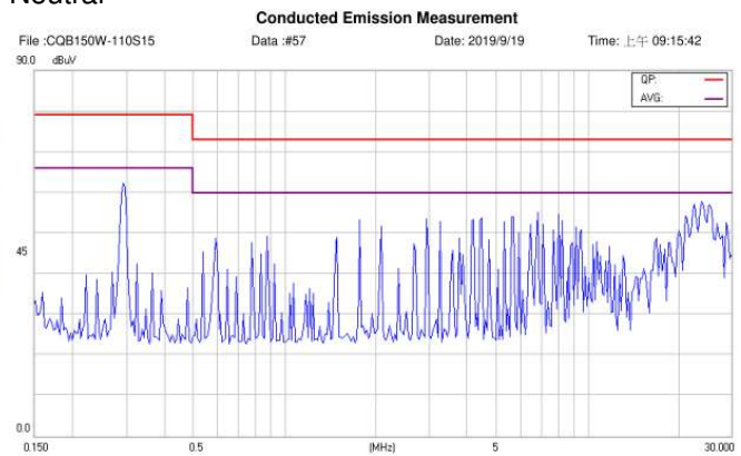
CQB150W-110S15-CMFC(D) Neutral
