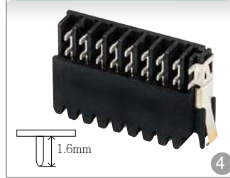
總線連接器/Bus connector BS-100
