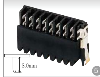
總線連接器/Bus connector BS-110
