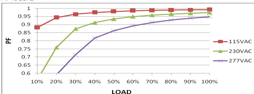
P.F vs LOAD
