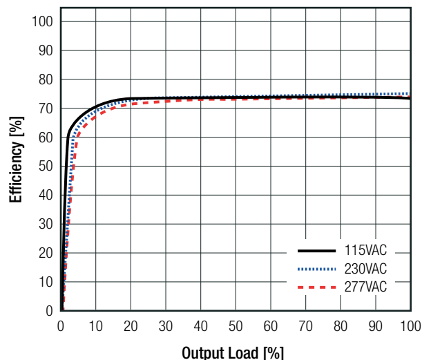
RAC03E-15SK/277
