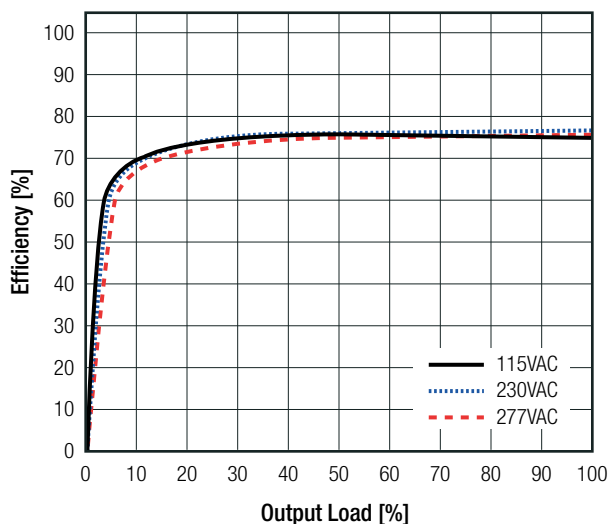
RAC03E-12SK/277 / RAC03E-24SK/277
