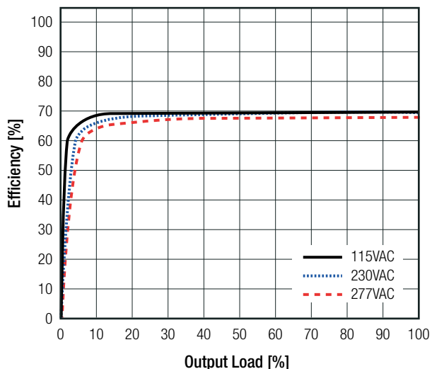
RAC03E-12SK/277 / RAC03E-24SK/277
