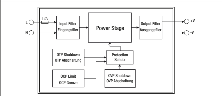
Fig. 2: Functional Diagram / Funktionsschema
