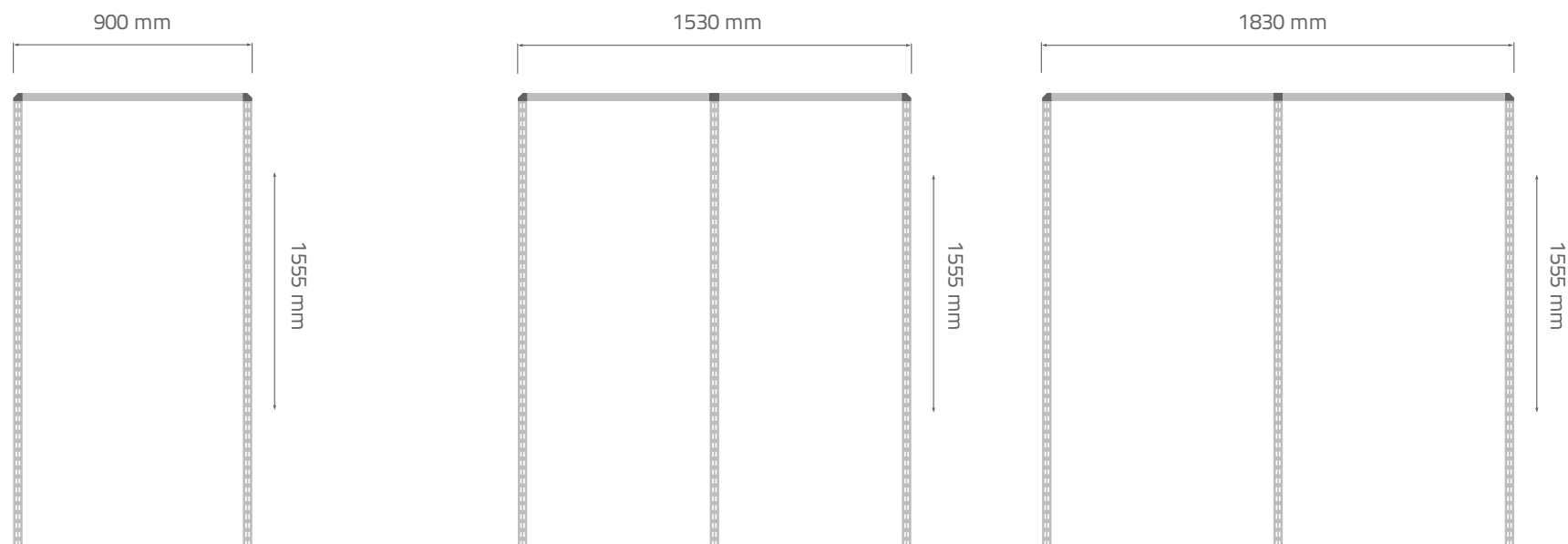
Perforierter vertikaler Rahmen - Maßtabelle
