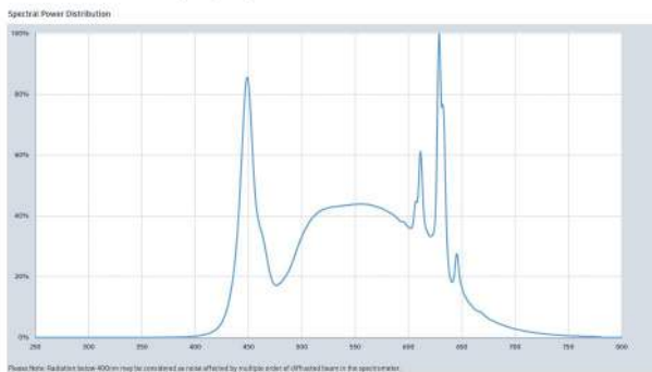
Samsung MPL 2835 LM281B+ PRO S90 VK, VL, S90, 5000K
